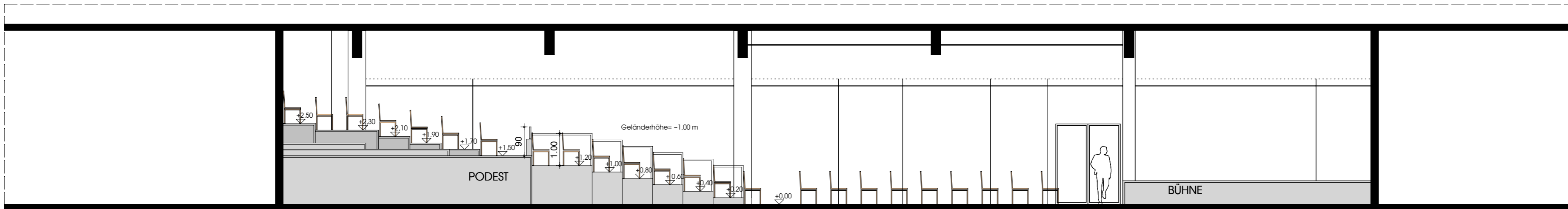
SCHNITT
